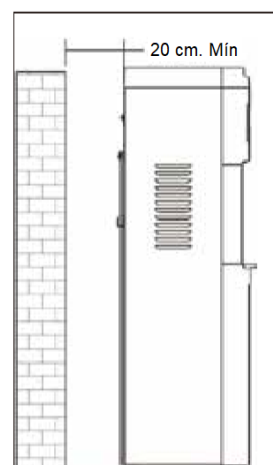
VISTA LATERAL
